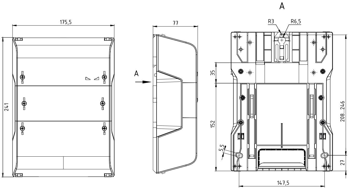
Рисунок 1 - Габаритные и установочные размеры
